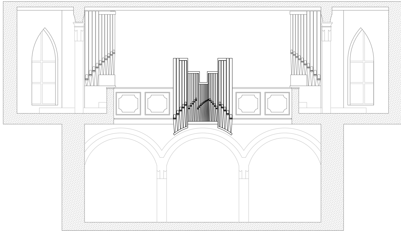
Frontansicht
